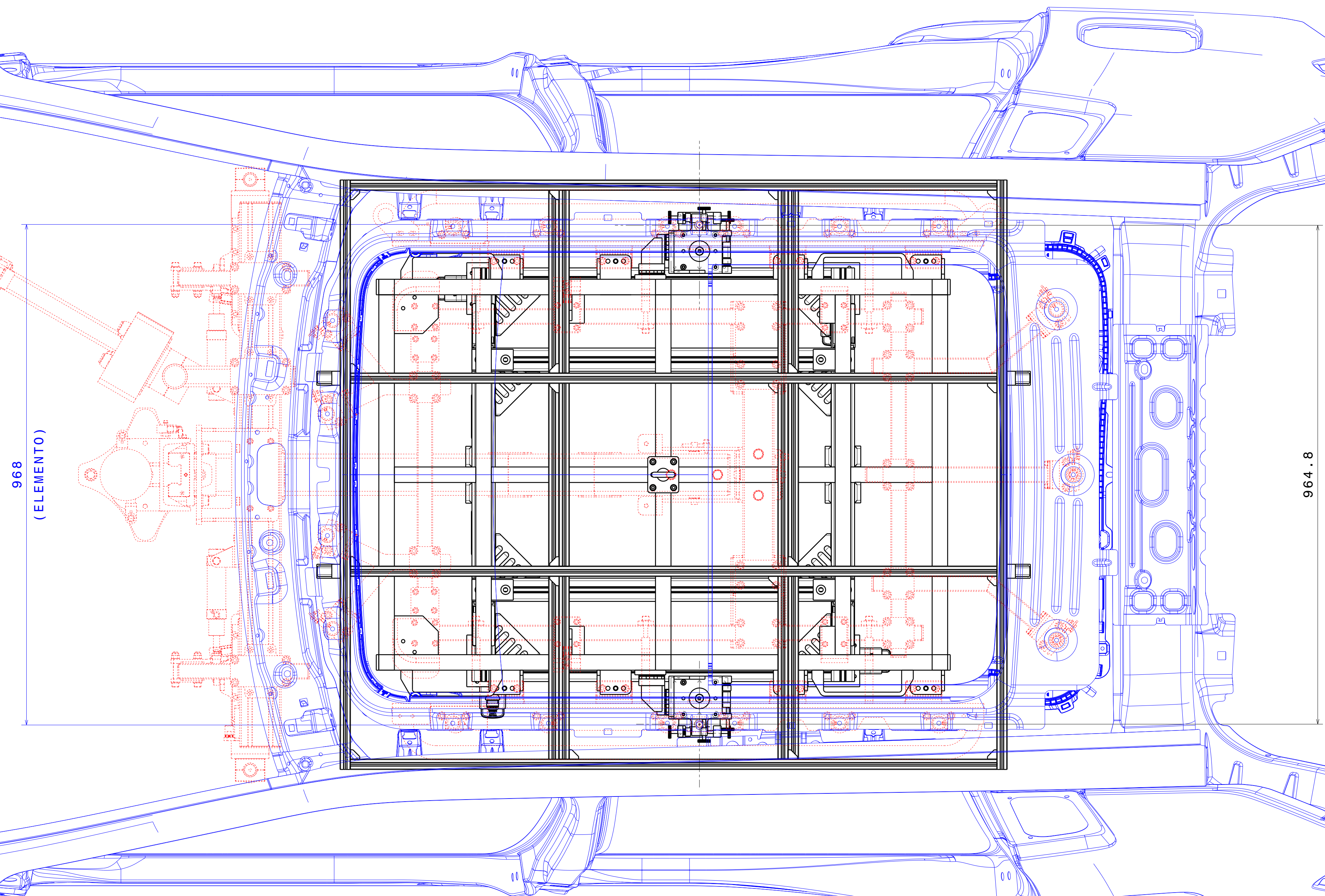
Vista frontale Scala: 1:5
