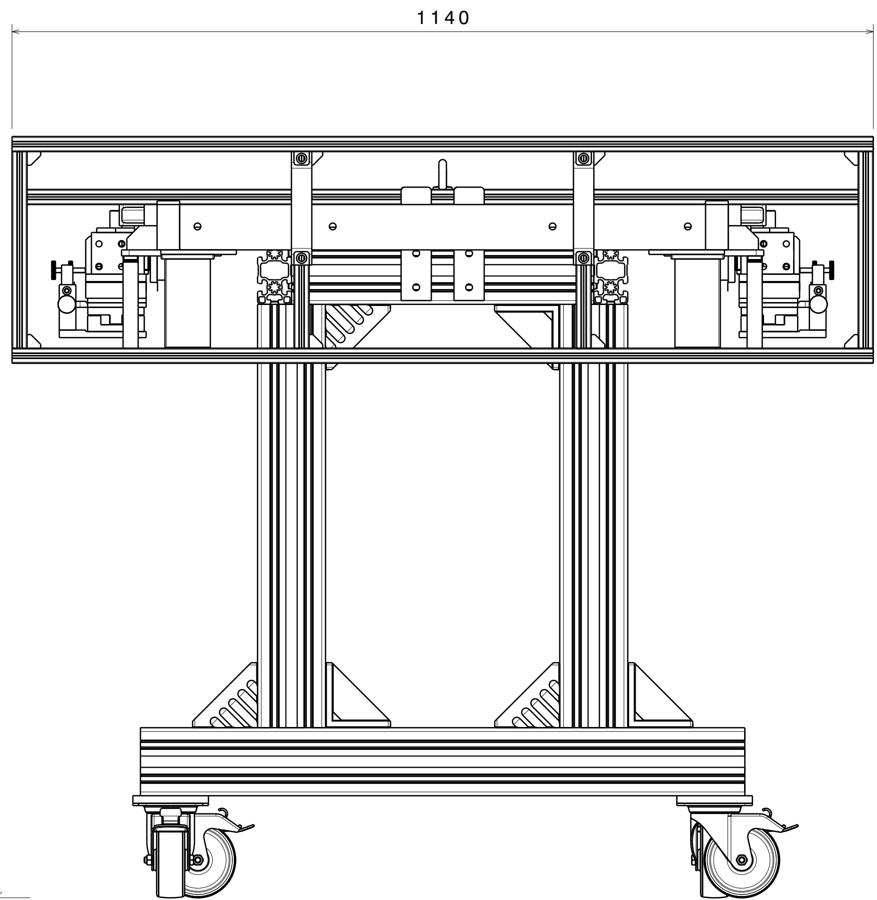
Vista ausiliaria A Scala: 1:5
