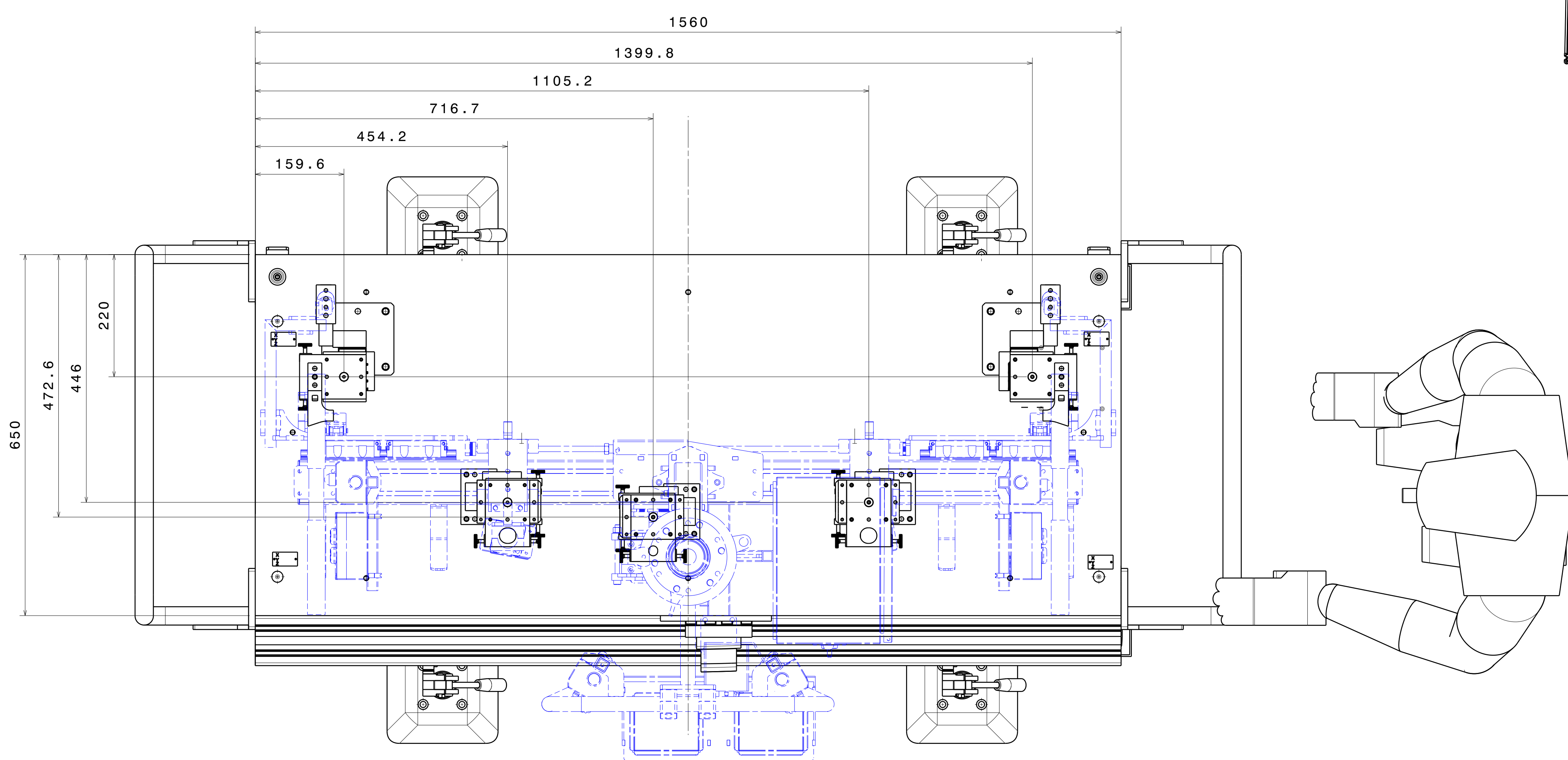
Vista dall'alto Scala: 1:5
