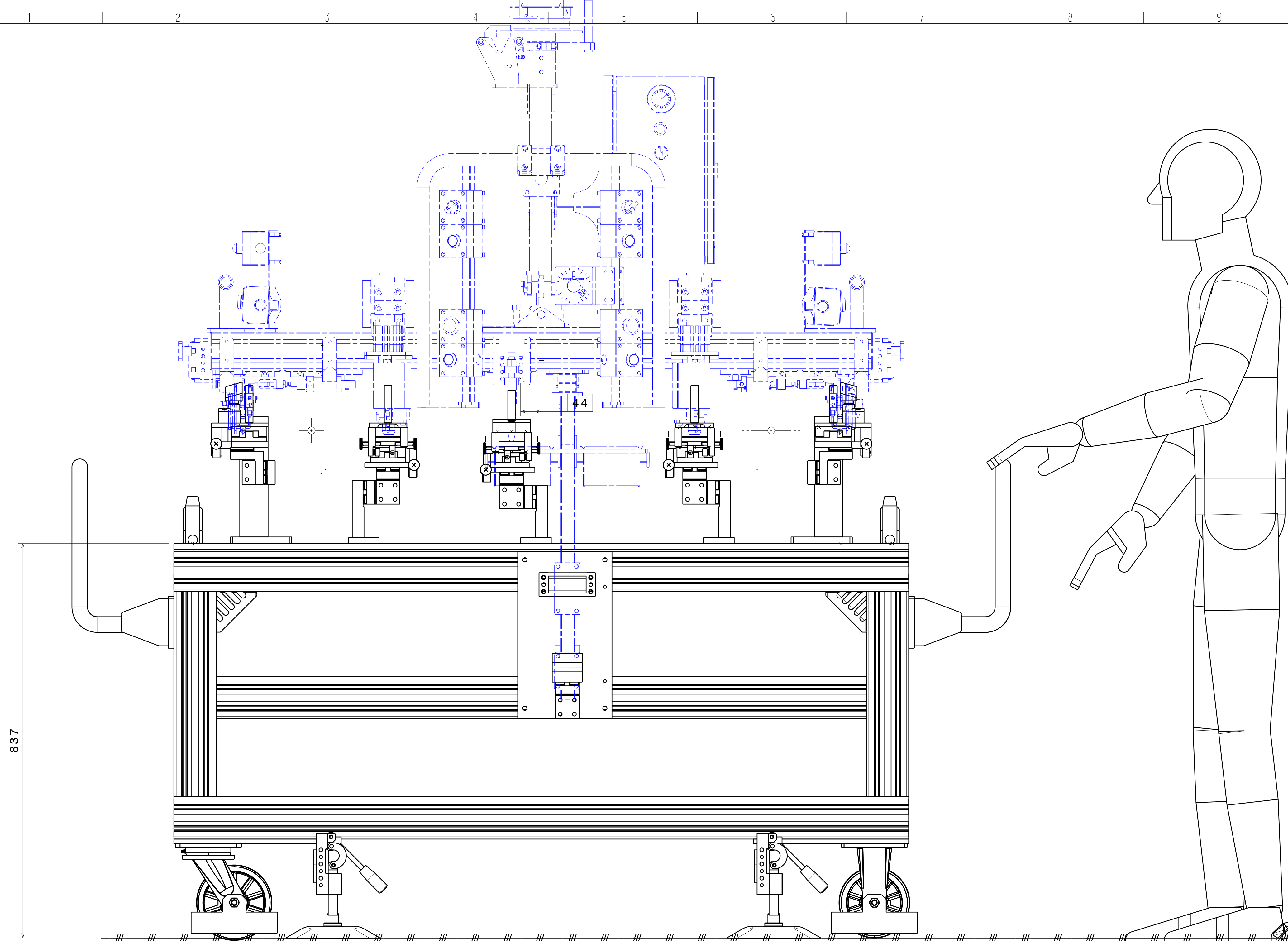
Vista frontale Scala: 1:5
