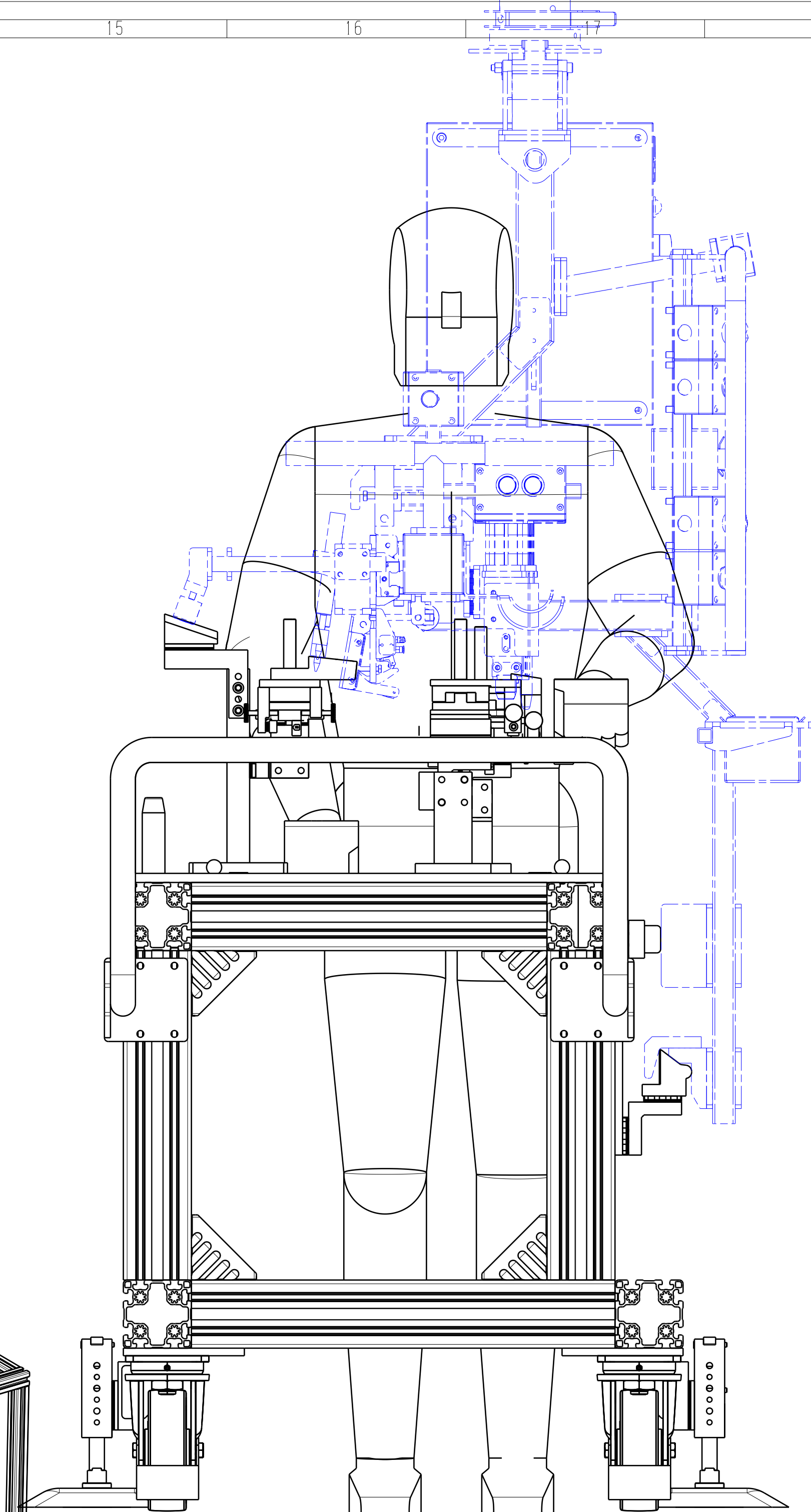
Vista da sinistra Scala: 1:5
